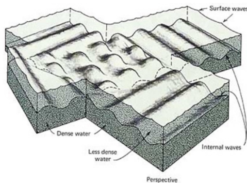
Figura 2: Mga panloob na alon at bahagi sa gitna ng dalawang magka-patong na tubig na may magkaibang kapal o bigat. Ang isa ay mabigat o siksik (sa ilalim na bahagi), ang isa naman ay hindi masyadong mabigat o siksik (sa taas na bahagi). ( Oceanography , Gross, p. 204.)
