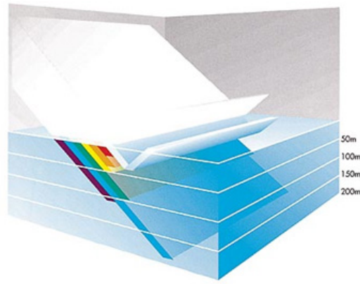
Figura 1: Nasa pagitan ng 3 at 30 porsiyentong sikat ng araw ang umaabot sa ibabaw ng dagat. Pagkaraa'y halos lahat ng pitong kulay ng tinatawag na Light Spectrum ay sunod-sunod na hinihigop ng tubig dagat sa unang 200 na metro, maliban na lamang sa kulay asul na liwanag. ( Oceans , Elder and Pernetta, p. 27.)
